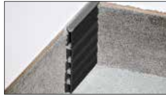
Schlüter®-DILEX-EZ 70 ist ein Entspannungs- und Zierprofil mit hinterschnittenen Seitenwänden aus Hart-PVC, mit einer Dehnungszone aus Weich-Kunststoff für den Einbau bei Mörtelverlegung. Die Verlängerungssegmente können entsprechend der Konstruktionshöhe abgetrennt werden. (Produktdatenblatt 4.2)
